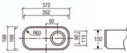
MIXA® H853 □ min. 300 mm U
