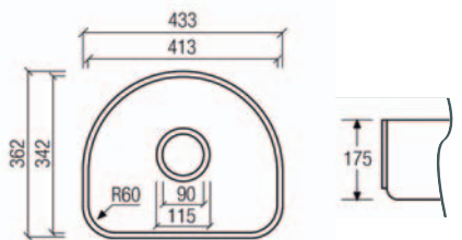
MIXA® H841 □ min. 400 mm #
