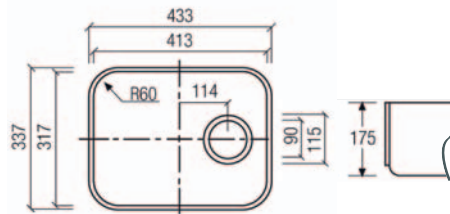
MIXA® H851 □ min. 400 mm #
